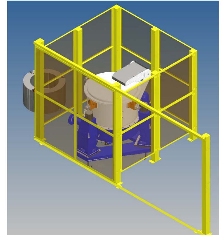
▲ Centrifuga Recuperadora de óleo modelo PCR 100% conforme NR-12
